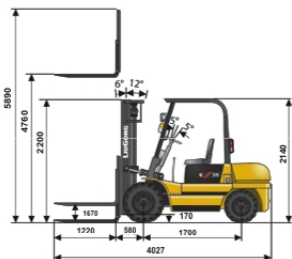
Dimensiones (mm)
