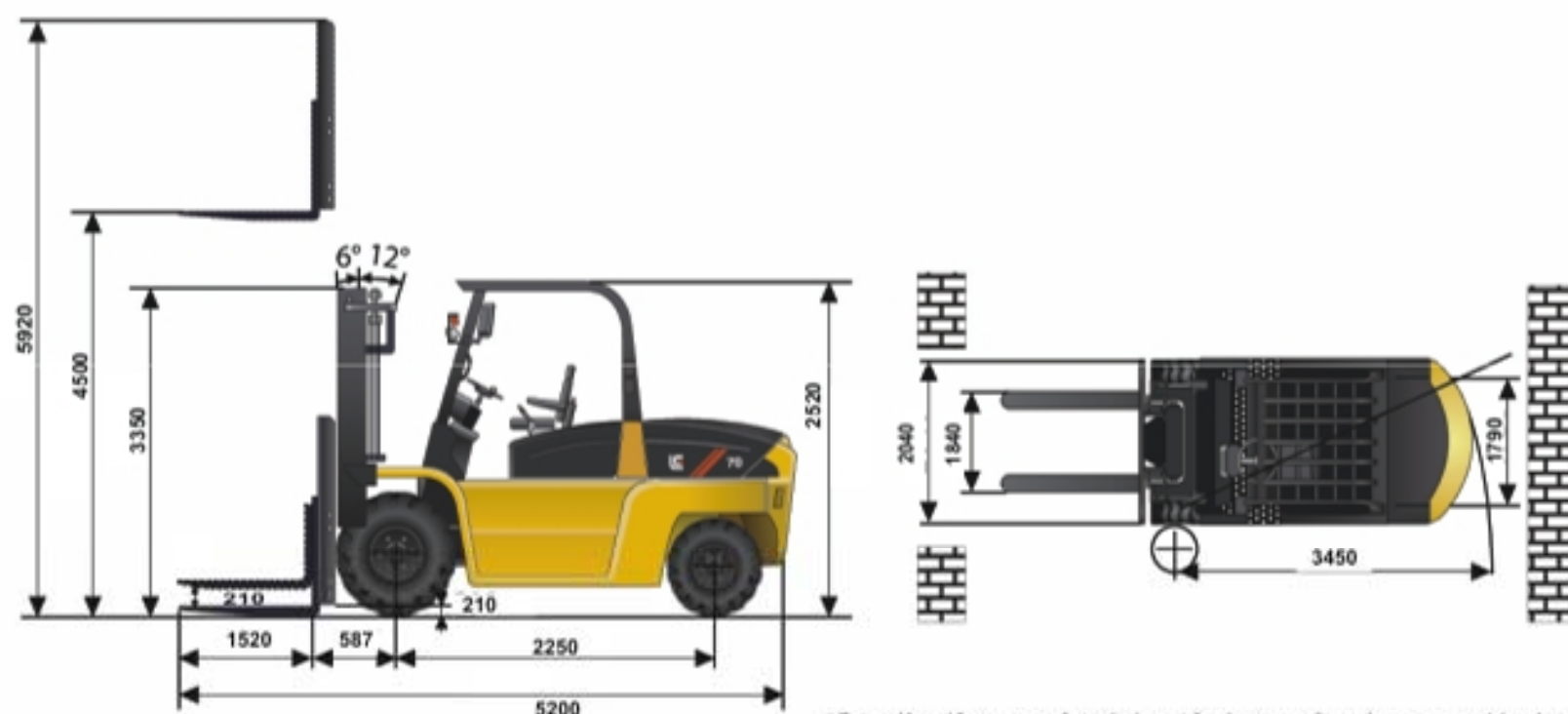
Dimensiones (mm)
